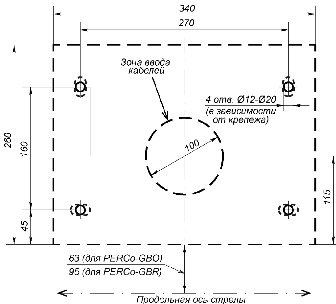
Рисунок 7. Разметка установочных отверстий шламбаума
