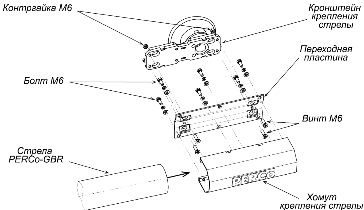
Рисунок 14. Монтаж стрелы PERCo-GBR
