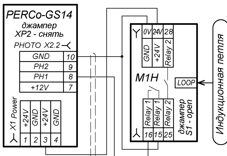
Рисунок 18. Схема подключения одноканального датчика M1H в качестве элемента безопасности и датчика проезда
