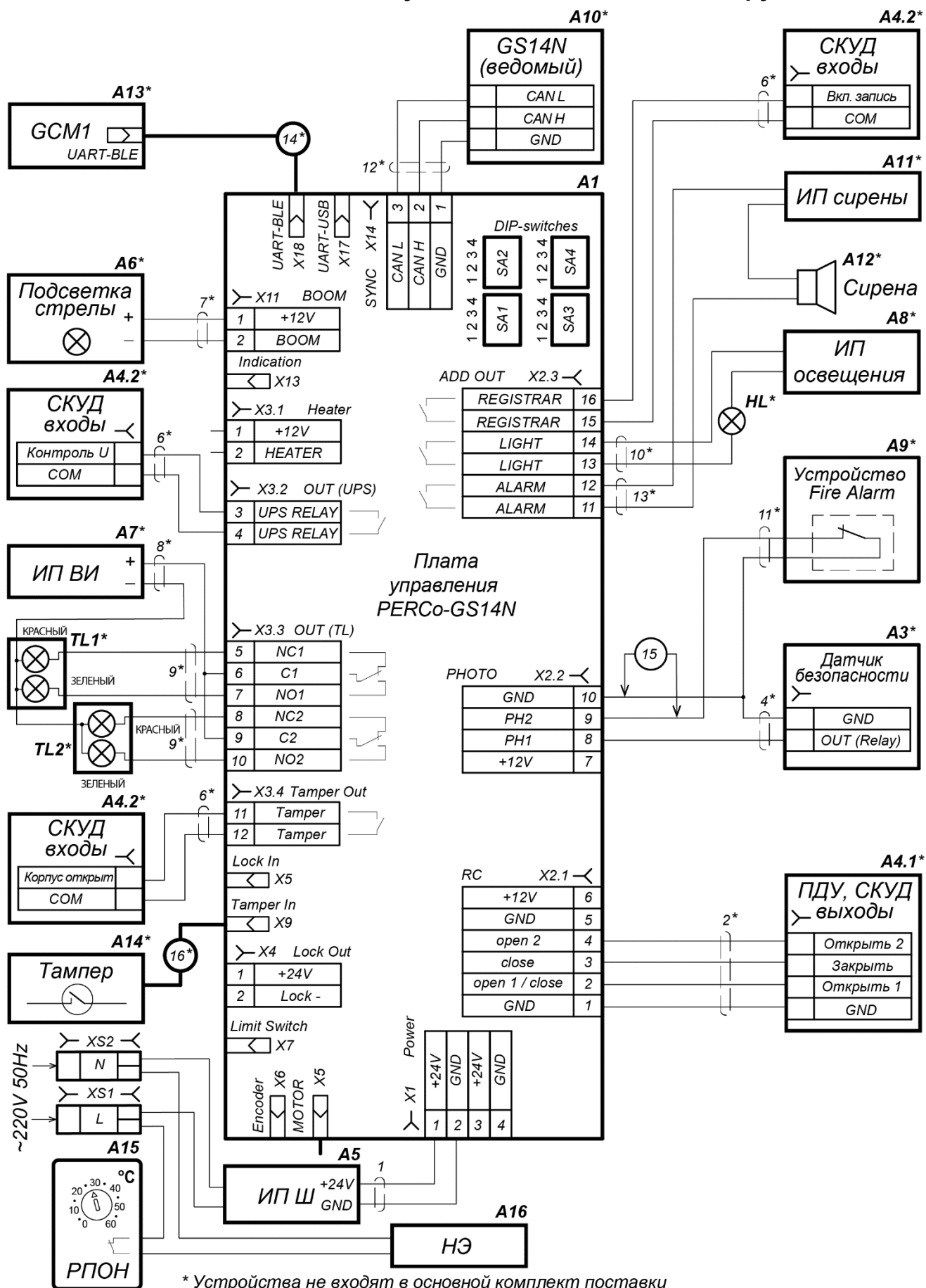
Рисунок 8. Схема подключения шлагбаума и доп. оборудования (перечень элементов см. в табл. 5)
