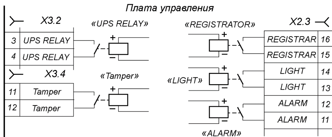
Рисунок 5. Выходные каскады для релейных выходов «ALARM», «LIGHT», «REGISTRATOR», «Тампер» и «UPS RELAY» платы управления
