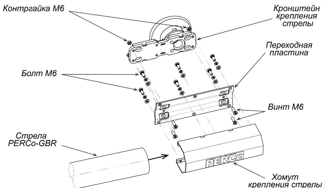
Рисунок 12. Монтаж стрелы PERCo-GBR
