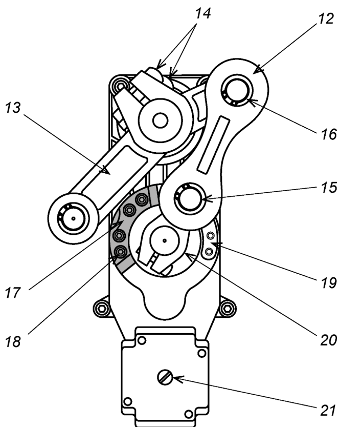
Рисунок 9. Порядок переустановки стрелы слагбаума
