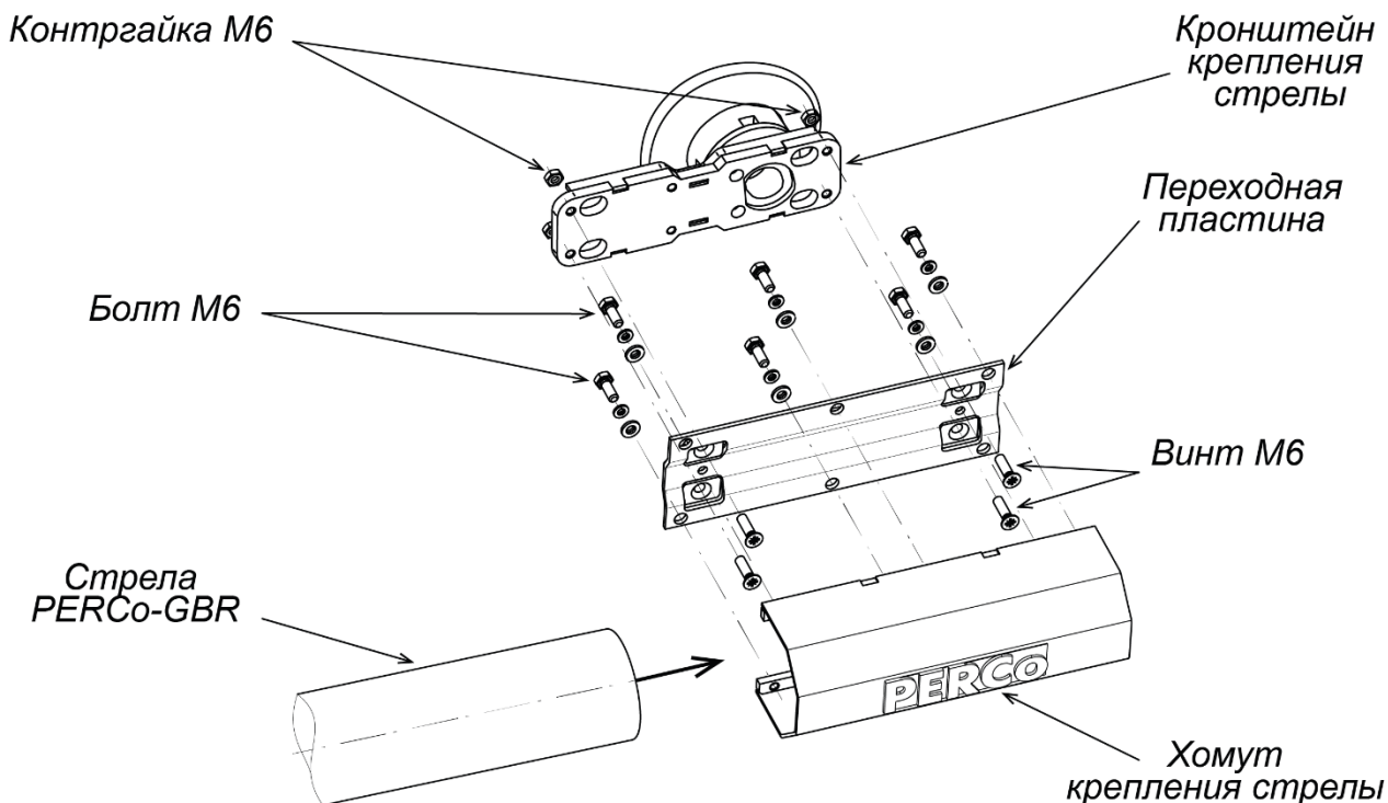
Рисунок 17. Монтаж стрелы PERCo-GBR
