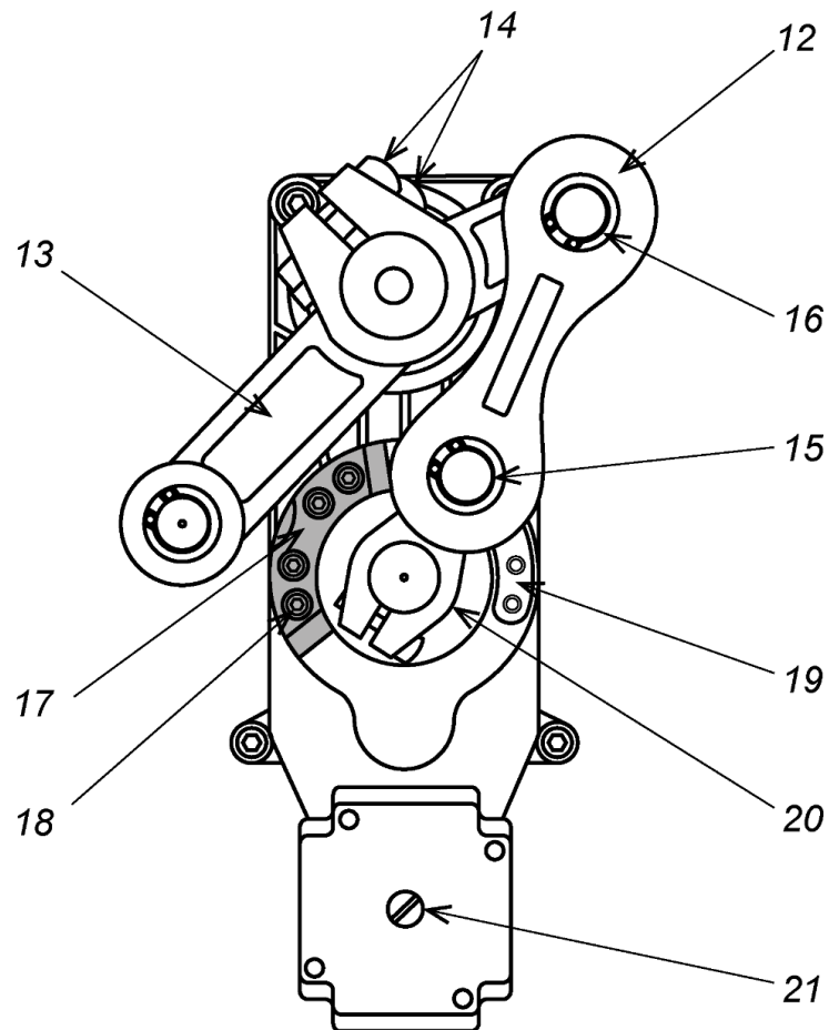
Рисунок 10. Порядок переустановки стрелы шлагбаума
