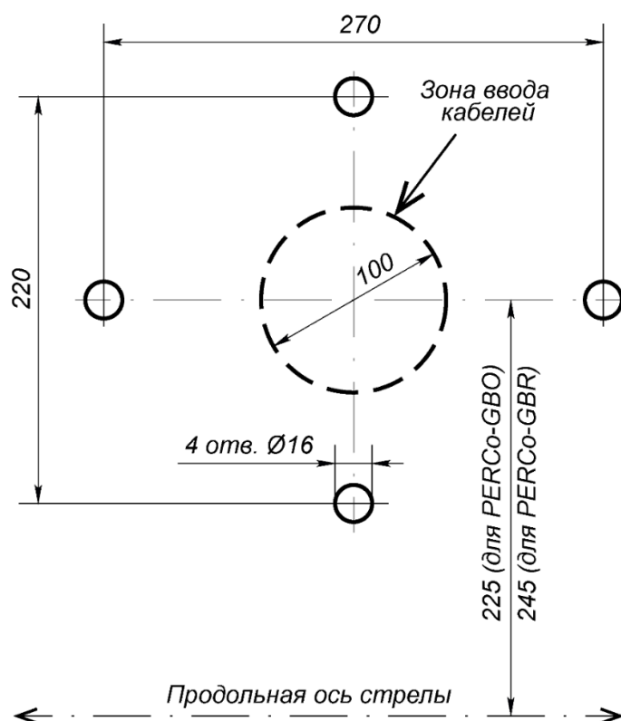
Рисунок 7. Разметка установочных отверстий шлагбаума
