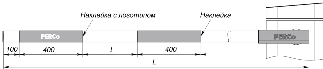
Рисунок 14. Наклеивание световозвращающих элементов на стрелу PERCo-GBR
