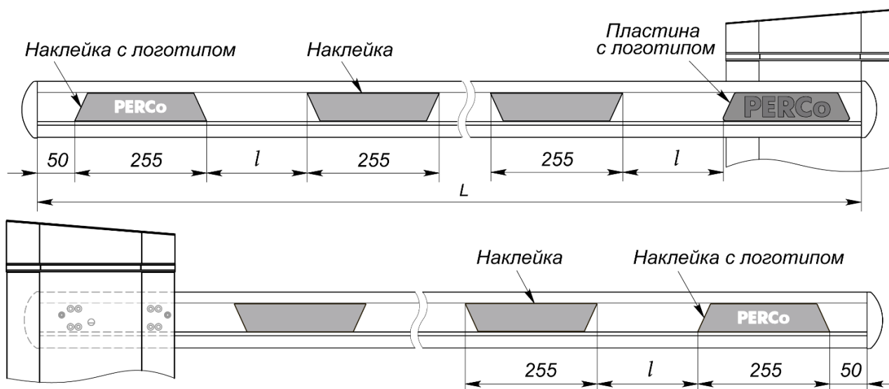
Рисунок 13. Наклеивание световозвращающих элементов на стрелу PERCo-GB0
