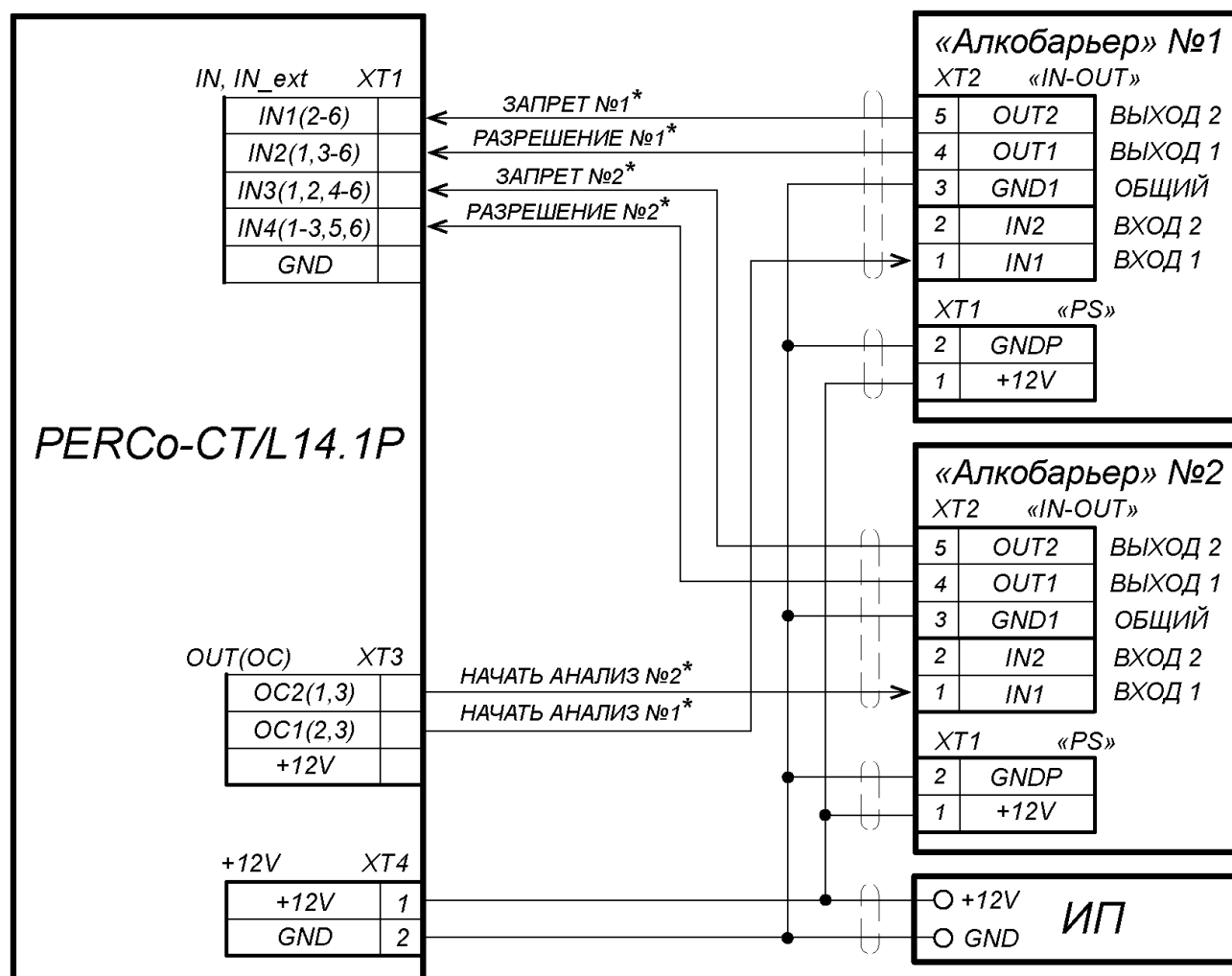
Рисунок 19. Схема подключения алкотестера «Динго В-02» (ООО СИМС-2)
