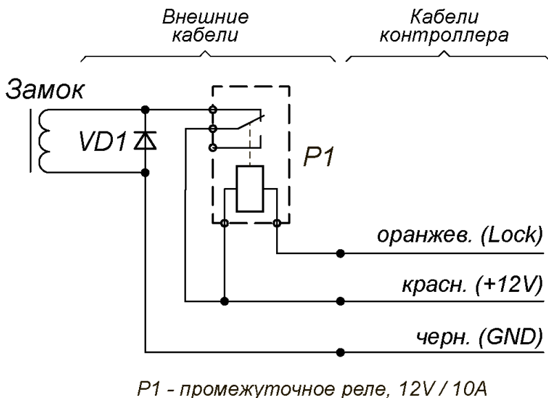
Рисунок 5. Схема подключения замка к контроллеру через промежуточное реле
