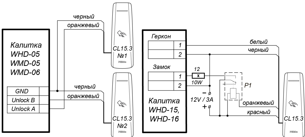
Рисунок 8. Схемы подключений калиток
