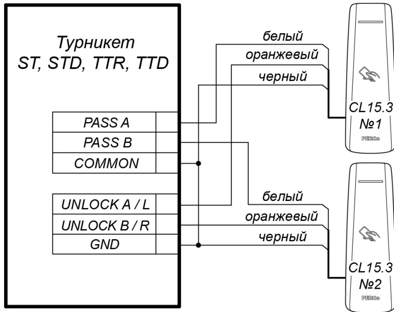
Рисунок 7. Схема подключений турникетов
